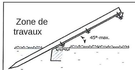
Schéma d'une barrière à sens unique ©BIOTOPE d'après English Nature (2001)
