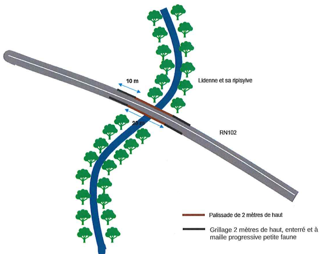
Schéma de principe des aménagements sur ouvrage hydraulique
