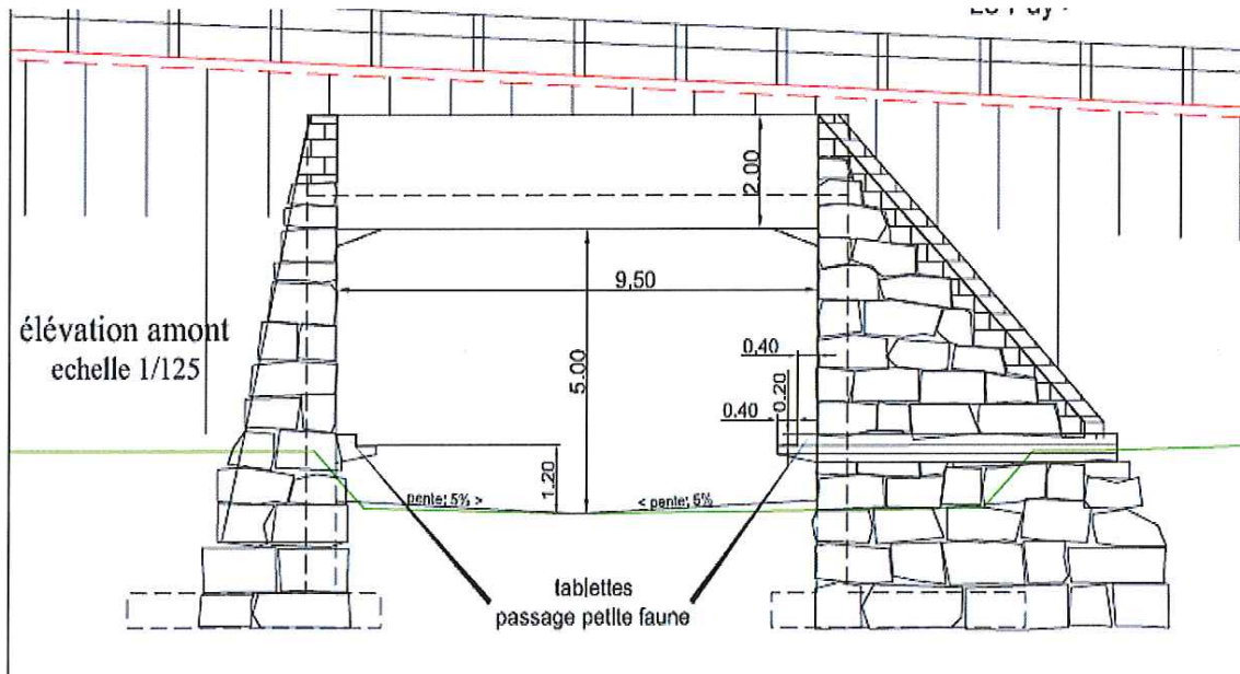
schéma de l'ouvrage de franchissement à créer
