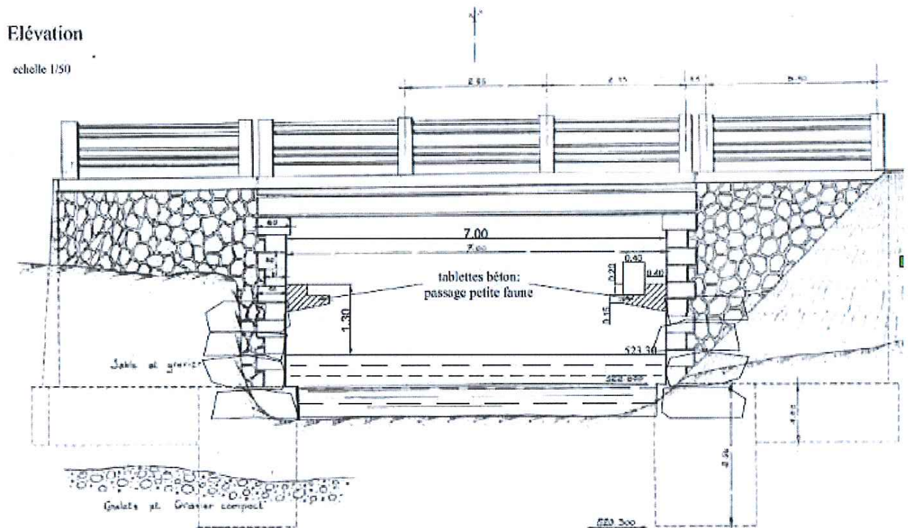
schéma de réhabilitation de l'ouvrage existant
